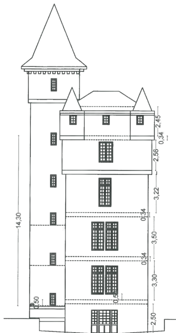
FACADE SUD-OUEST
